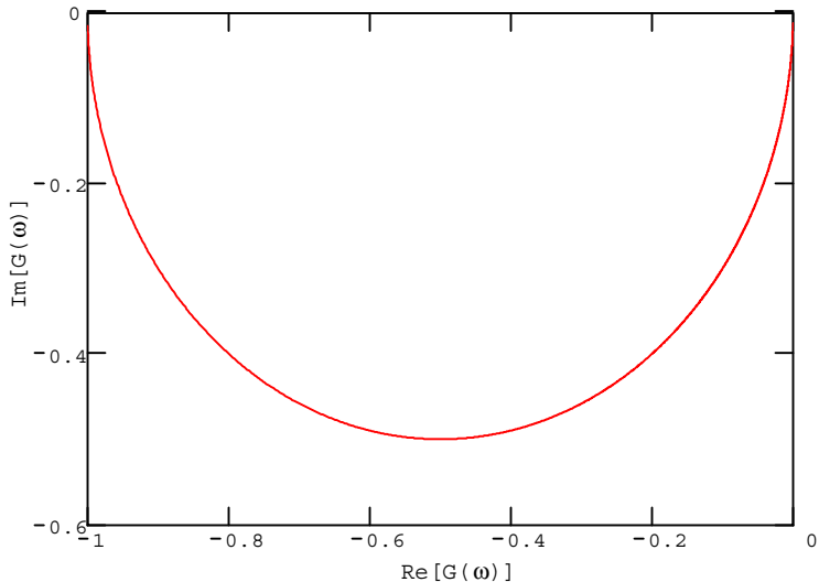
Nyquist plot per un circuito passa-basso
