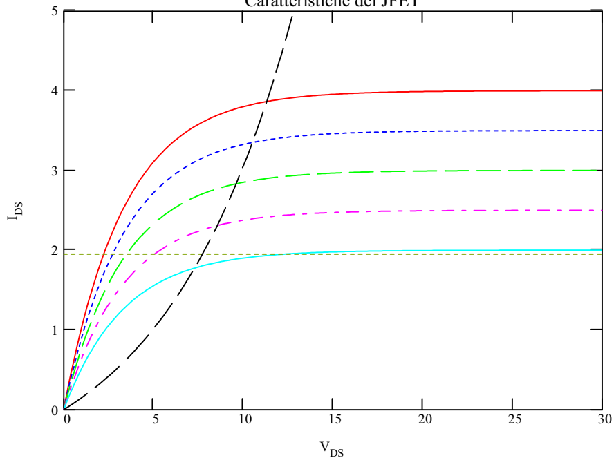
Caratteristiche del JFET
