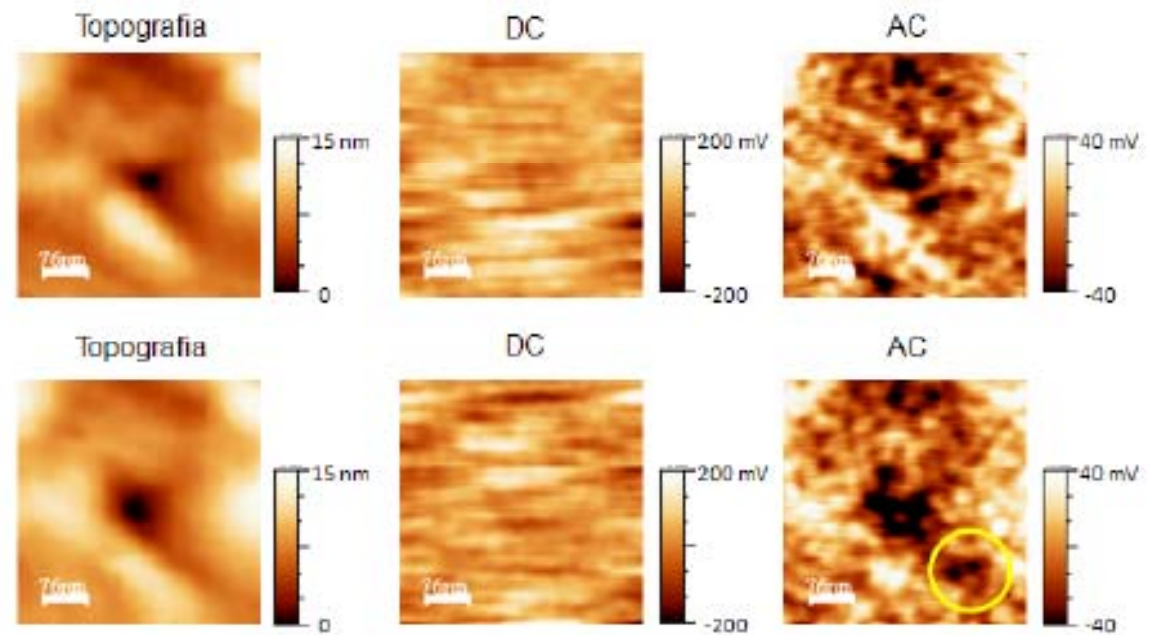
Figura 6.11: Mappe acquisite con lo SNOM su una zona di un campione di PMA4/PMMA 20b80 dove è stata effettuata una nanoscrittura. In alto: mappe prima della scrittura. In basso: mappe dopo la scrittura. L'area di scansione è 400 \text{ nm} \times 400 \text{ nm} con una risoluzione di 128 \times 128 pixels; l'impulso ha potenza P=10\text{mW} e durata \Delta t=2 \text{ ms} . La posizione della nanoscrittura è indicata con un cerchio nella mappa AC in basso a destra.
